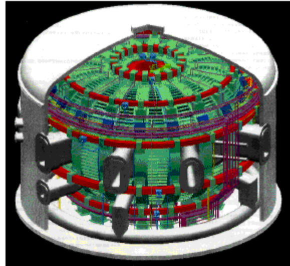
JT60-SA
